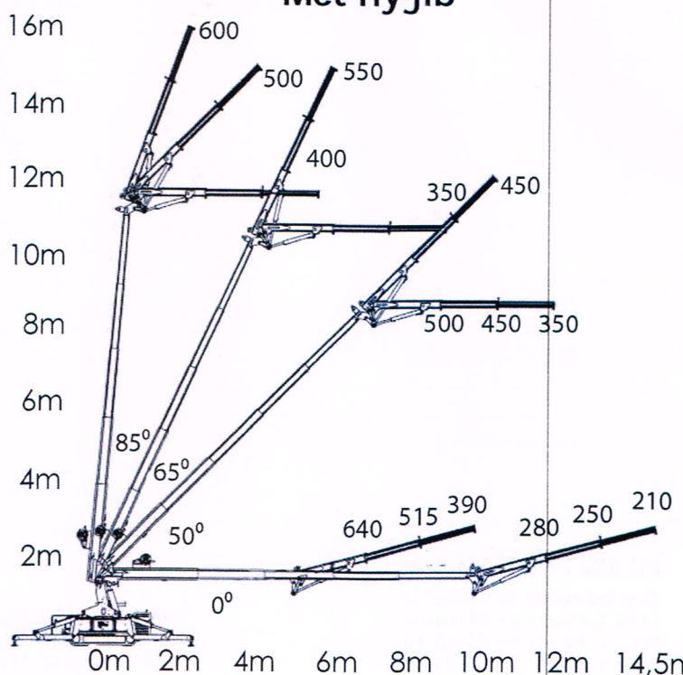
Met fly-jib
